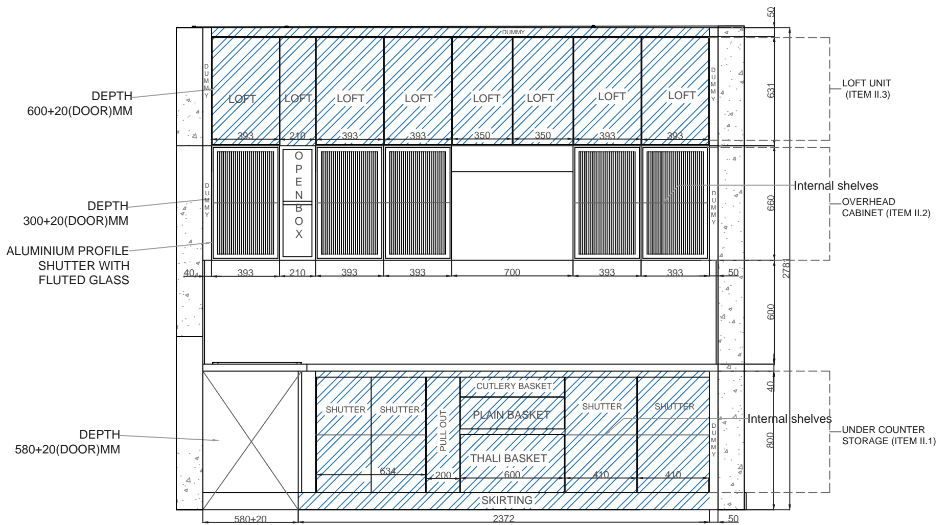
Elevation A
